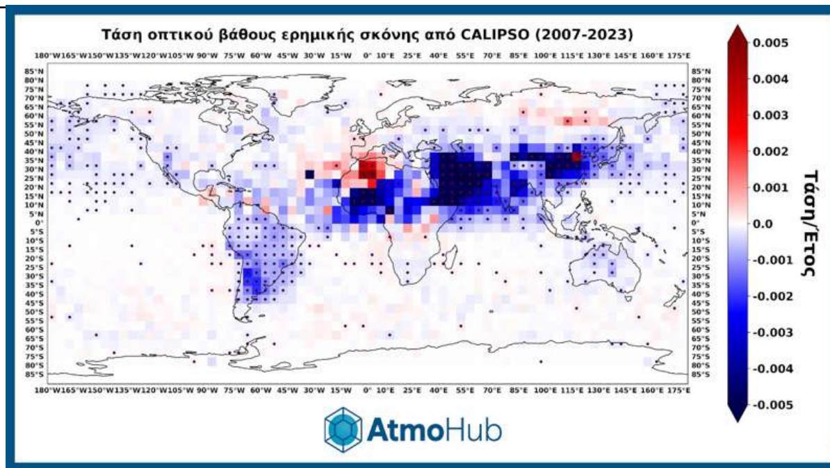
Εικόνα 1: Τάση οπτικού βάθους ερημικής σκόνης (ποσότητα ανάλογη των συγκεντρώσεων) σε διάφορες περιοχές του πλανήτη από τον δορυφόρο CALIPSO, για την χρονική περίοδο 2007-2023.
